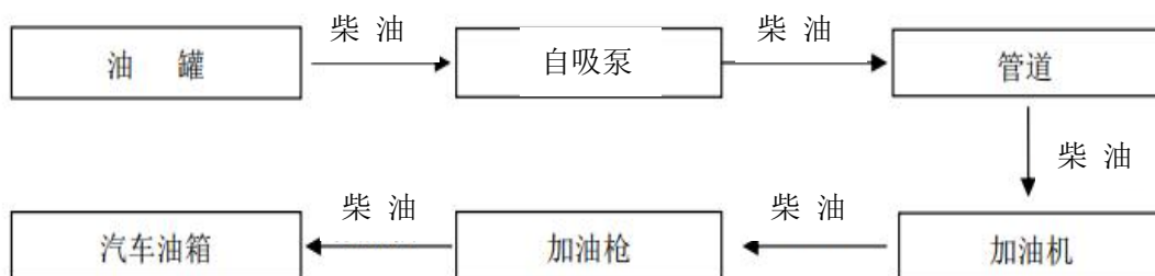
图 2-6 柴油加油工艺流程框图
