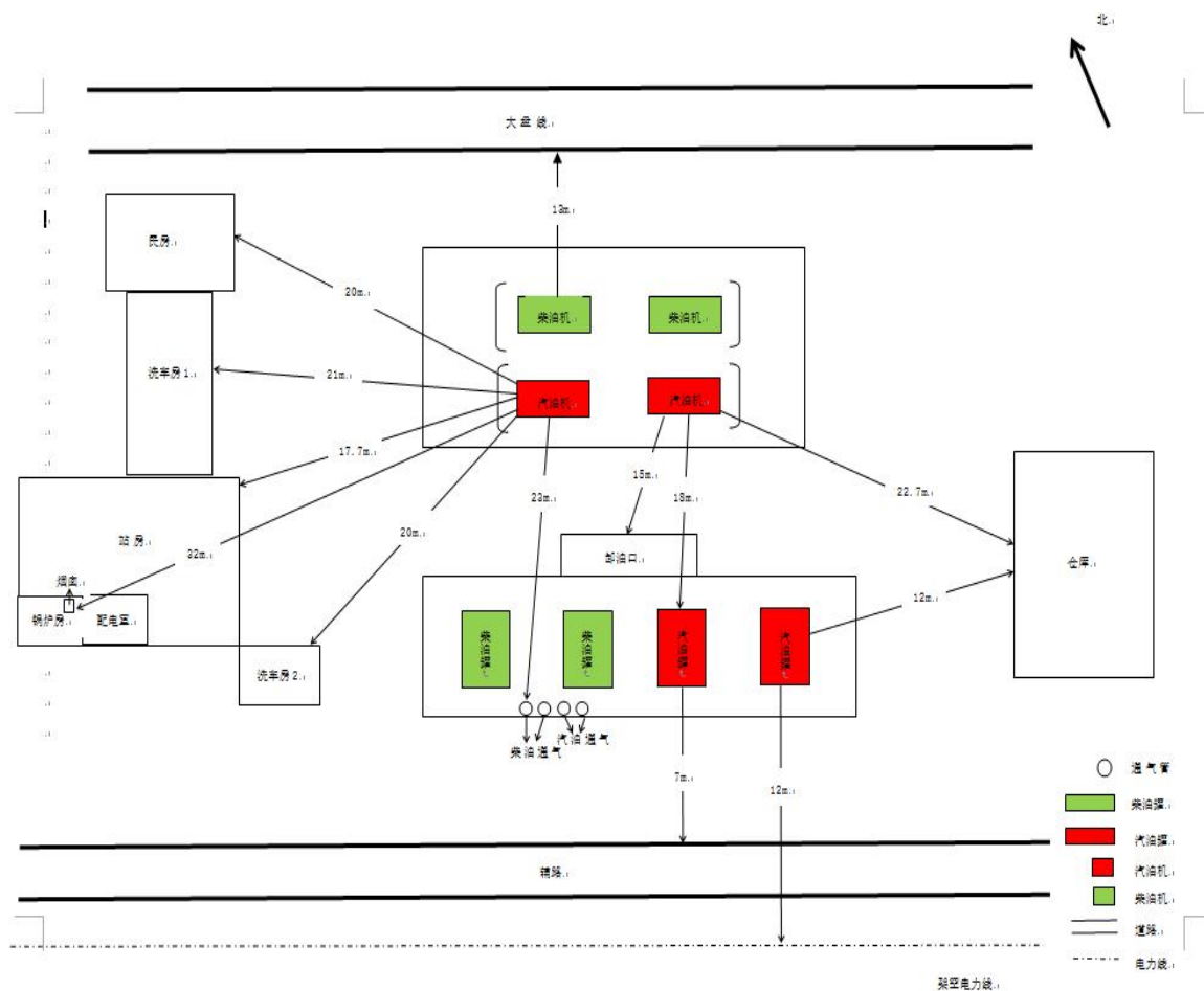
2-2 平面布置示意图
